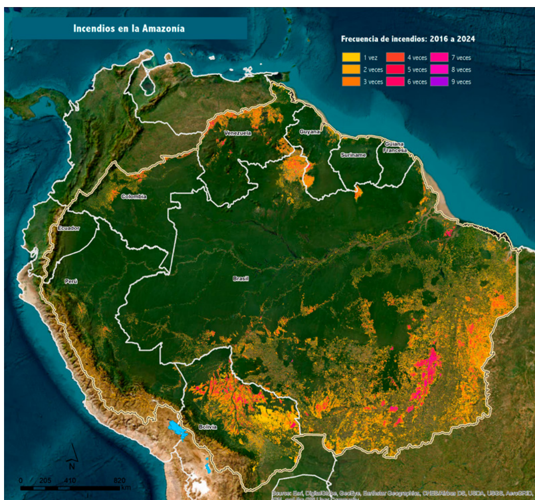
Figura 6. Áreas afectadas por quemas e incendios en la Amazonía: 2016 - 2024.
