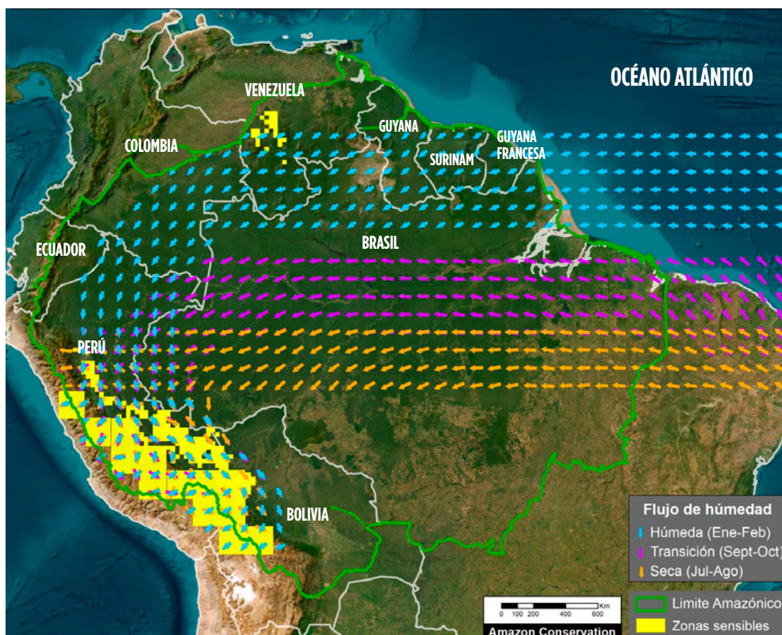
Figura 3. Flujos de humedad en la Amazonía con las zonas sensibles. Datos: ERA5, ACA/MAAP
